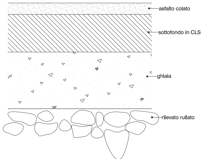
Pavimentazione esterna in asfalto su terrapieno
