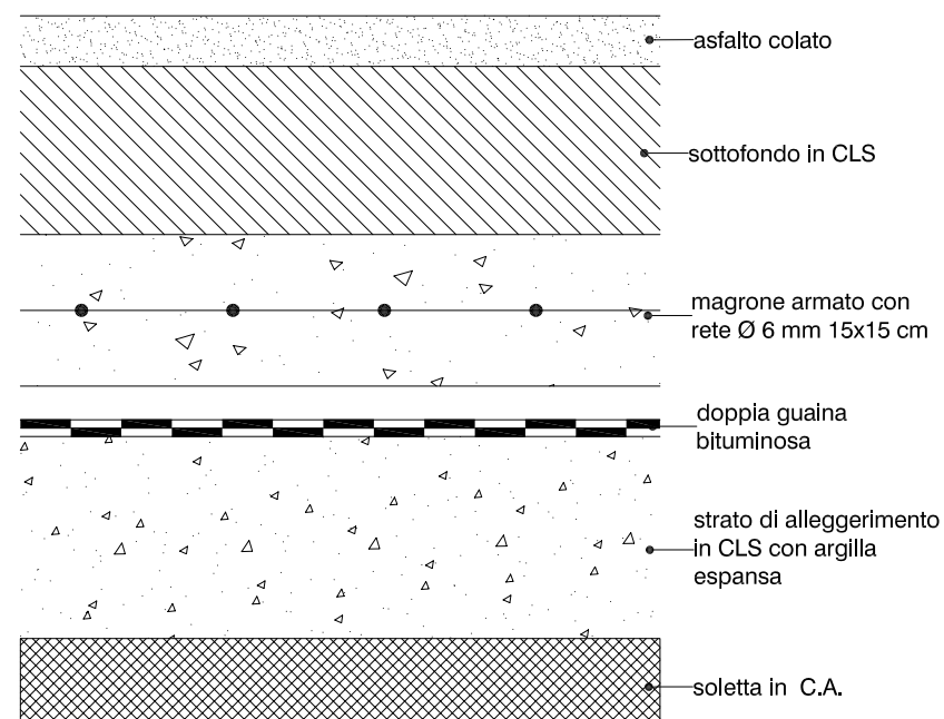
Pavimentazione esterna in asfalto su soletta
