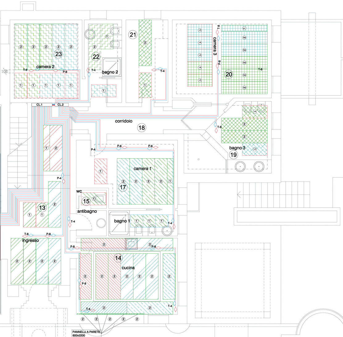
PANNELLI A PARETE 600x2200
