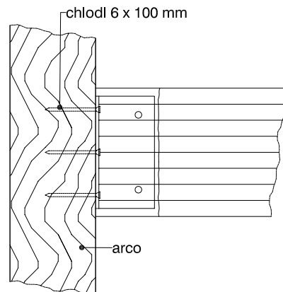
sezione A - A
