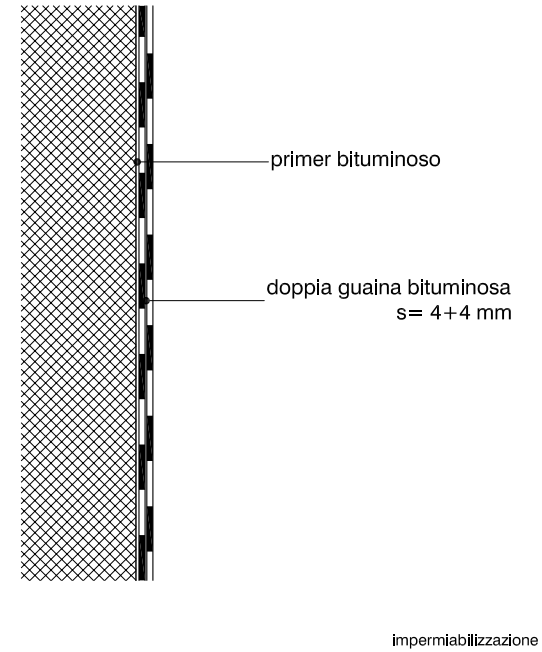
Dettaglio costruttivo di una parete in cemento impermeabilizzata con uno strato di primer bituminoso e una doppia guaina bituminosa ( sp = 4 + 4 mm).
