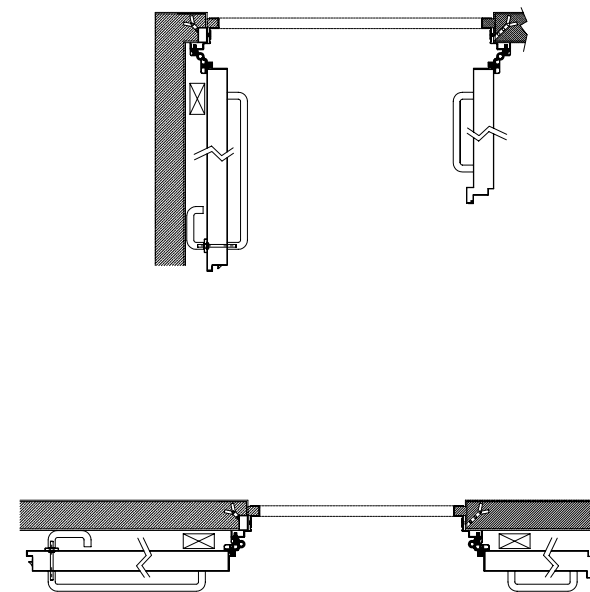
scala 1: 50 modalità di apertura
