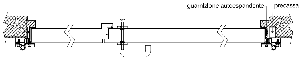
scala 1: 10 sezione B - B
