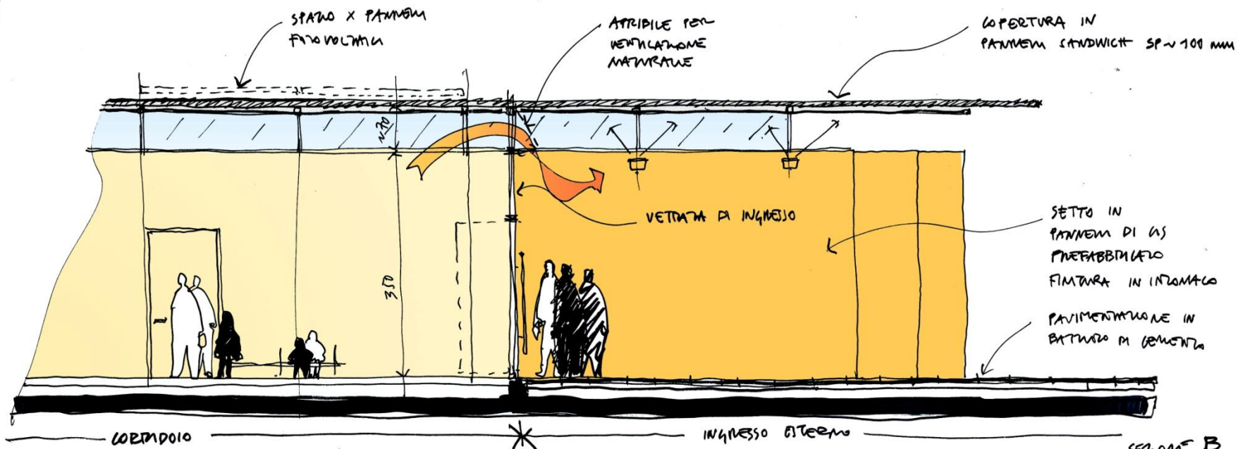
SEZIONE B SCALA 1:50
